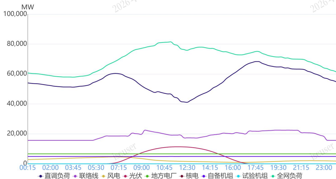
图 1 10月29日负荷及电源出力预测情况
