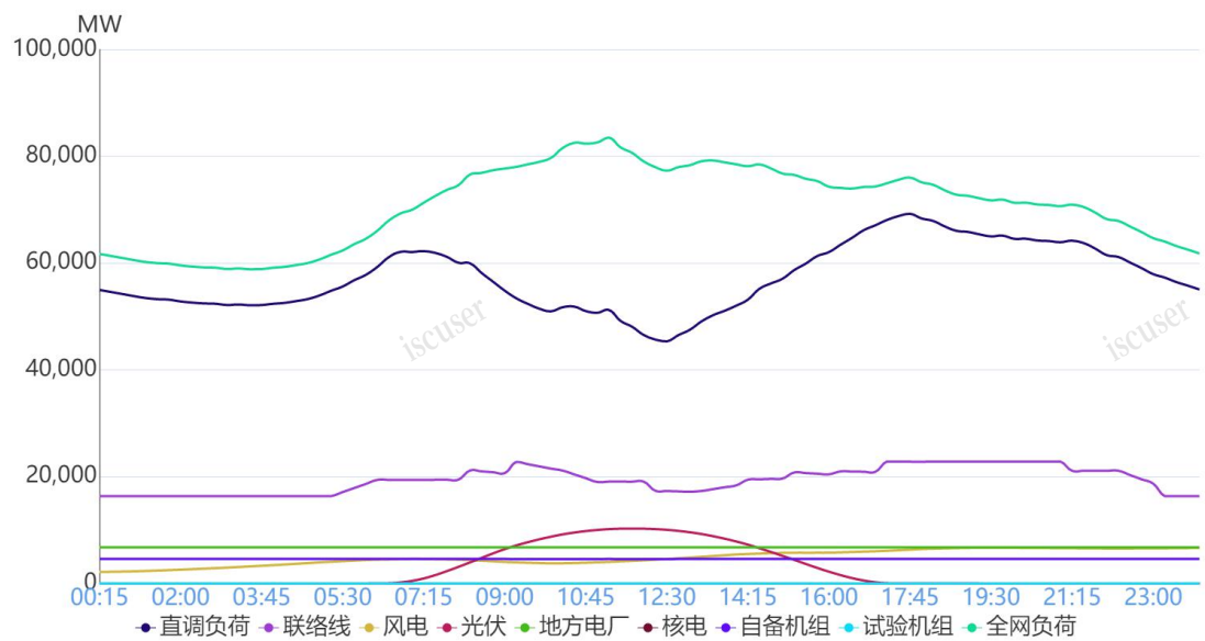
图 1 11 月 1 日负荷及电源出力预测情况
