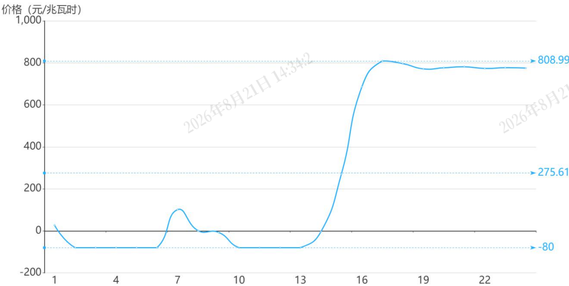
图 3 11 月 4 日实时市场用电侧价格
