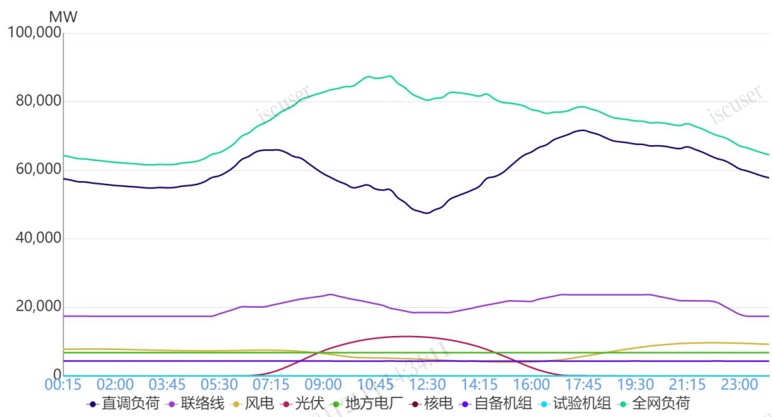
图2 11月7日负荷及电源出力预测情况
