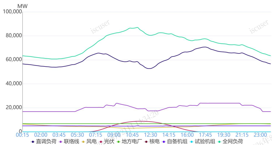
图 1 11月9日负荷及电源出力预测情况
