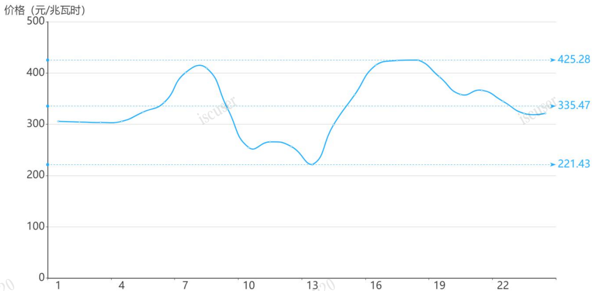
图2 11月9日日前市场用电侧价格
