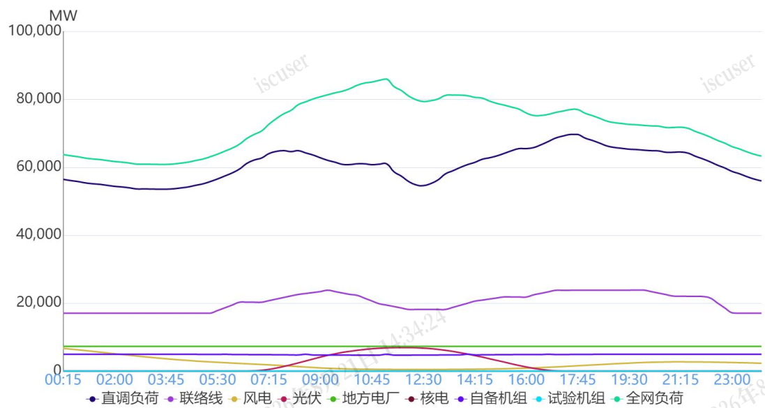
图 1 11月10日负荷及电源出力预测情况
