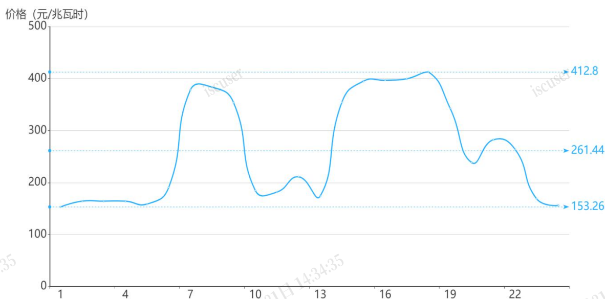
图 2 11 月 12 日日前市场用电侧价格
