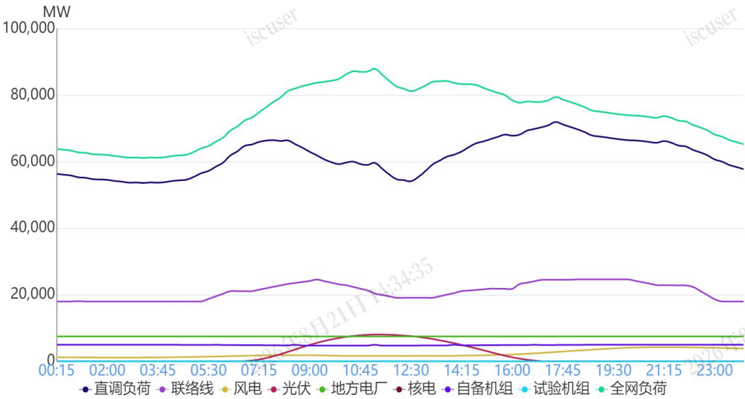
图 1 11月12日负荷及电源出力预测情况
