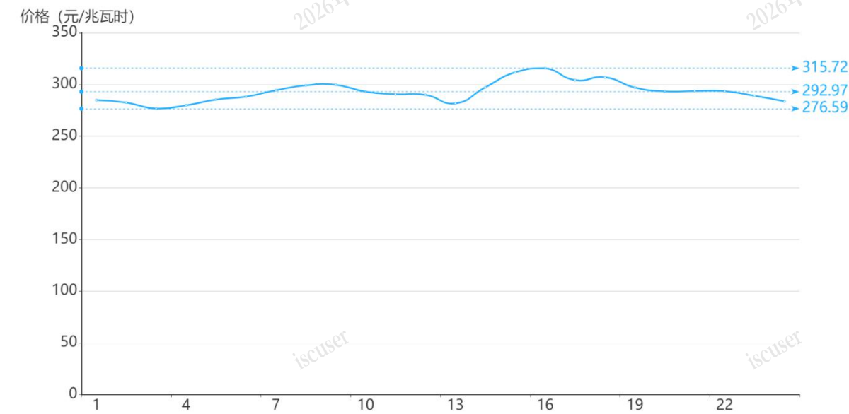
图 3 11 月 15 日实时市场用电侧价格
