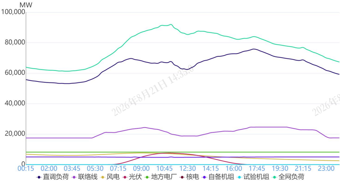
图 1 11月18日负荷及电源出力预测情况
