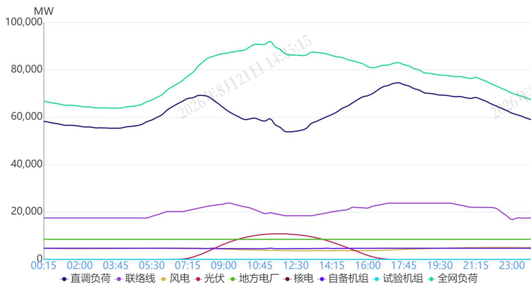
图 1 11月22日负荷及电源出力预测情况
