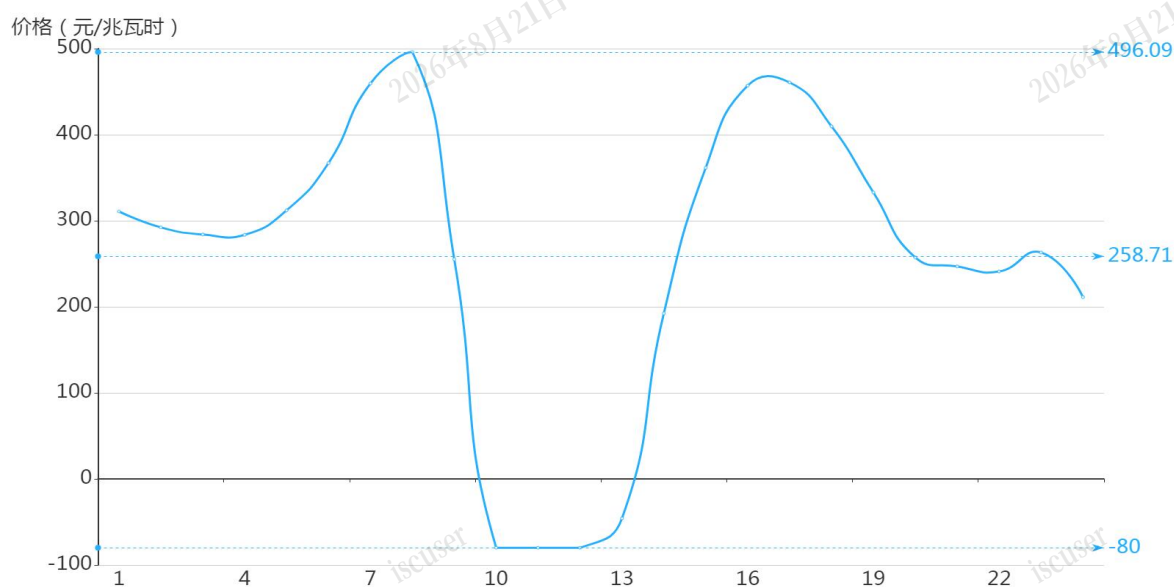
图4 11月22日实时市场用电侧价格
