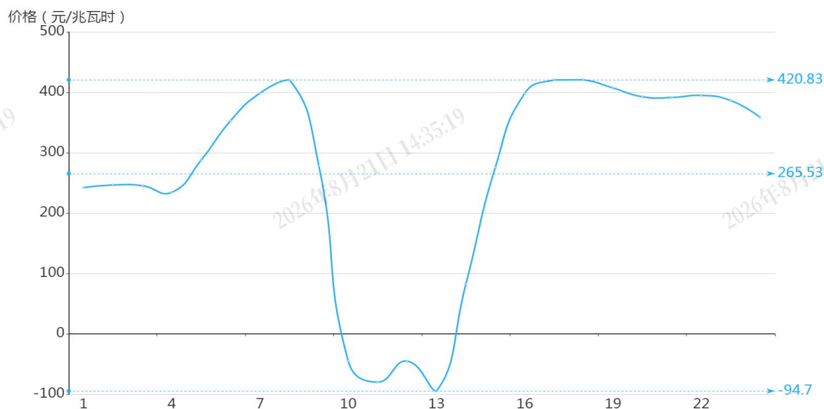
图 2 11月 23 日日市场用电侧价格
