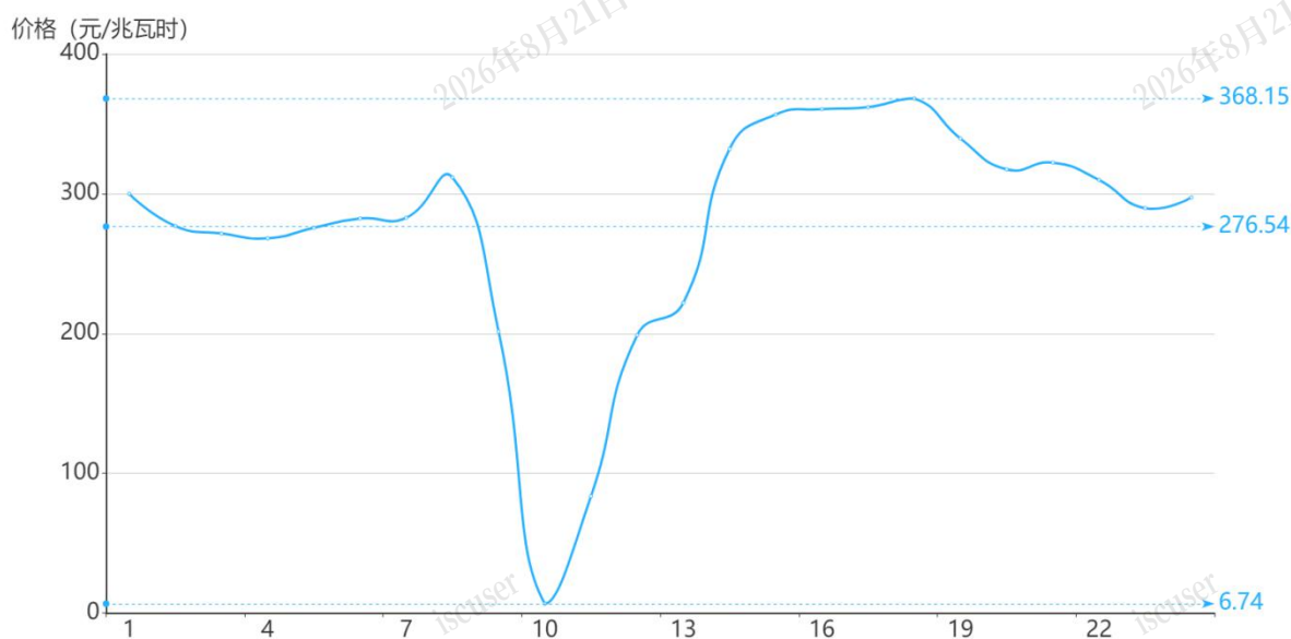
图3 11月24日实时市场用电侧价格
