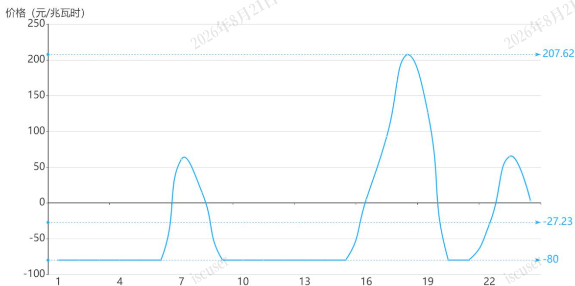
图3 11月26日实时市场用电侧价格
