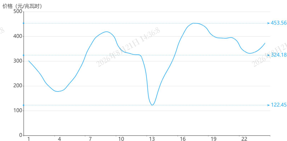
图 3 12 月 5 日实时市场用电侧价格
