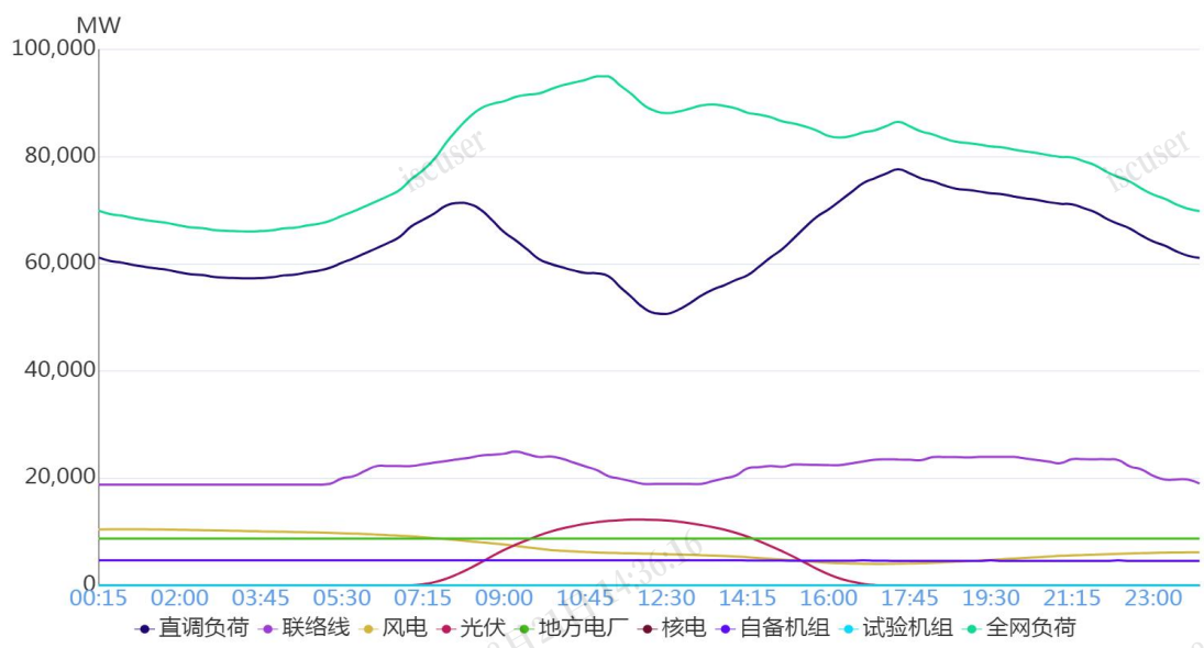
图 1 12月8日负荷及电源出力预测情况
