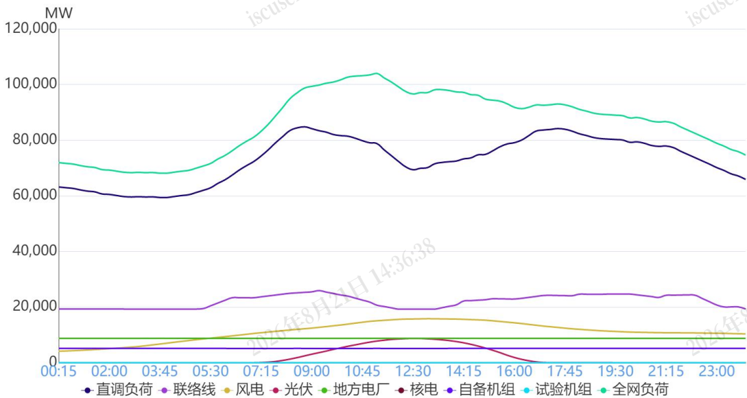
图 1 12月13日负荷及电源出力预测情况
