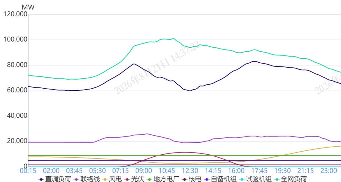
图 1 12月20日负荷及电源出力预测情况
