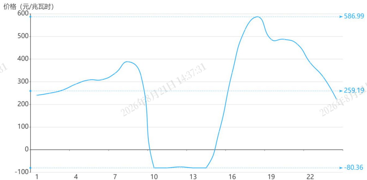
图2 12月22日日前市场用电侧价格
