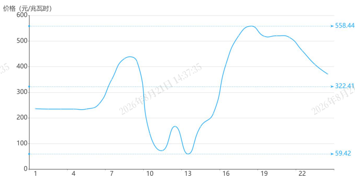
图2 12月23日日前市场用电侧价格
