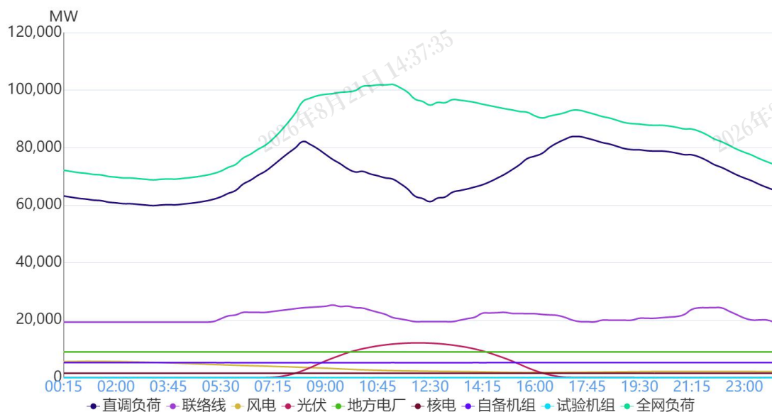
图1 12月23日负荷及电源出力预测情况
