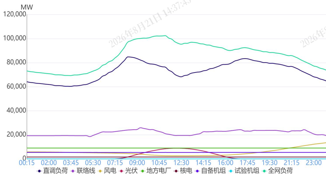
图 1 12月25日负荷及电源出力预测情况
