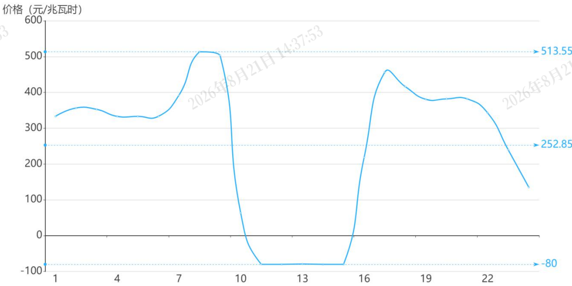
图 2 12 月 27 日日前市场用电侧价格
