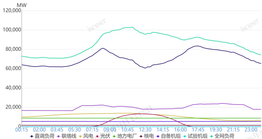
图 1 1月9日负荷及电源出力预测情况
