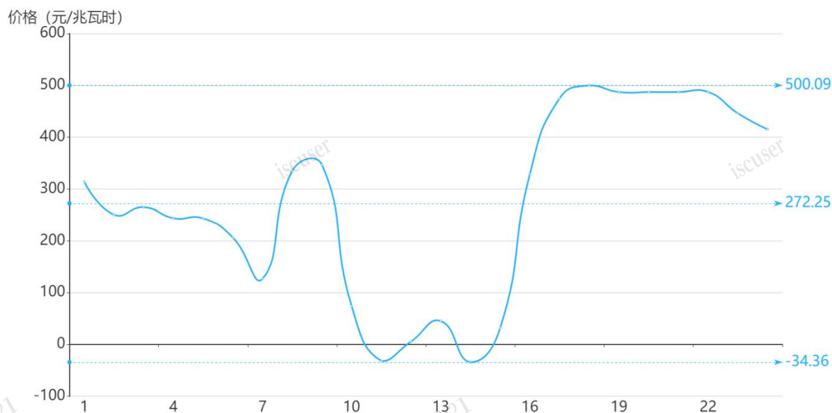
图2 1月9日日前市场用电侧价格
