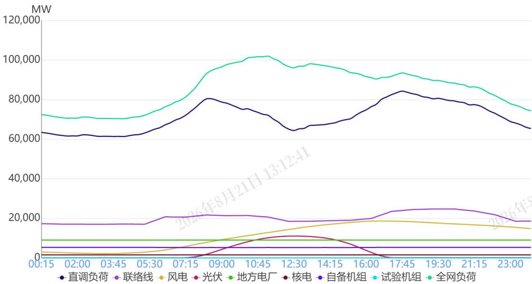
图 1 1月14日负荷及电源出力预测情况
