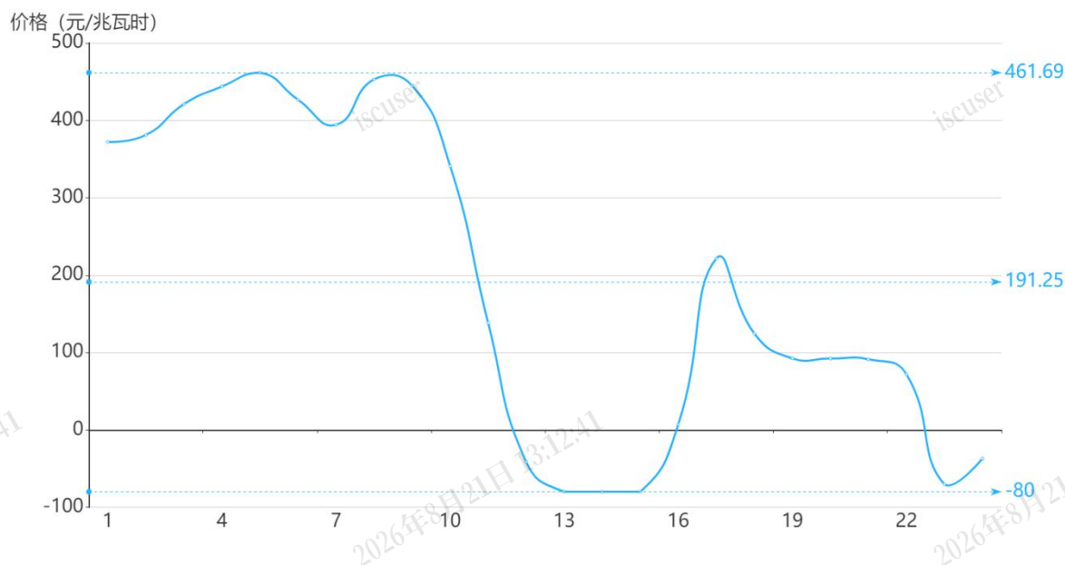
图2 1月14日日前市场用电侧价格
