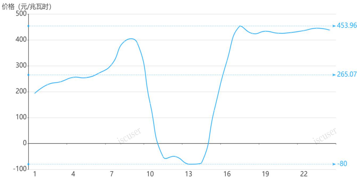
图 3 1 月 16 日实时市场用电侧价格
