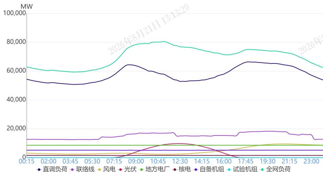
图 1 1月24日负荷及电源出力预测情况
