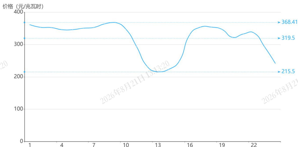
图 2 1 月 24 日日前市场用电侧价格
