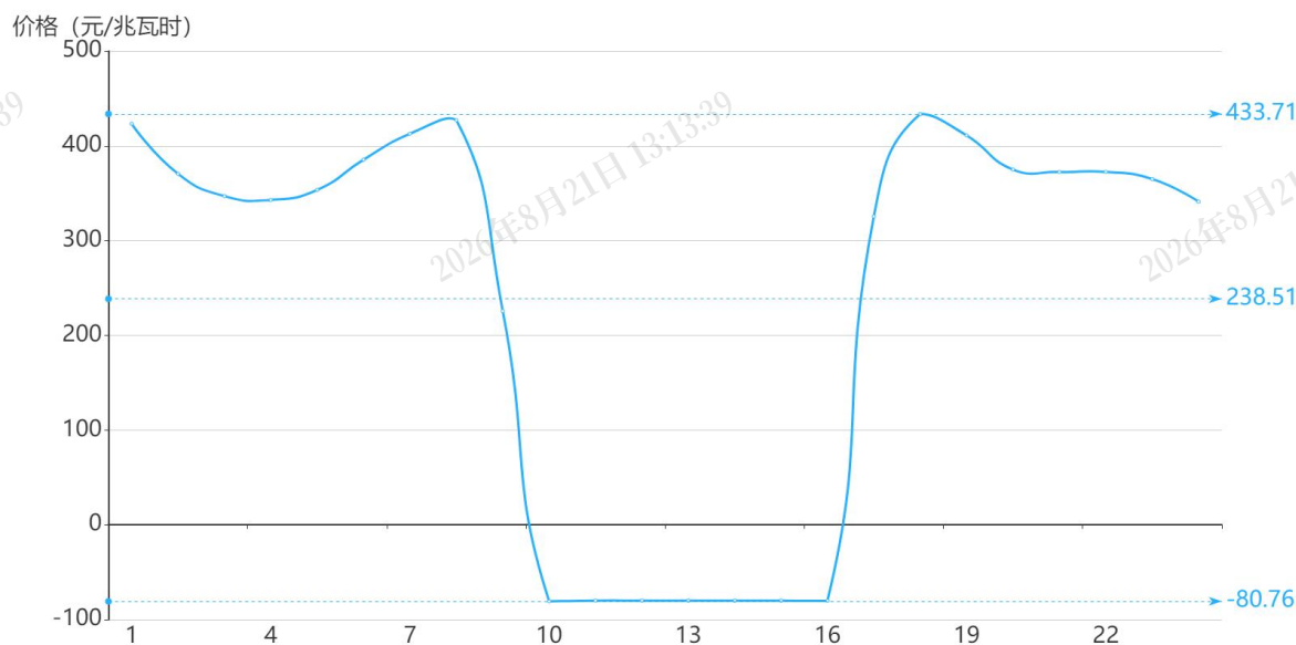
图 2 1 月 29 日日前市场用电侧价格
