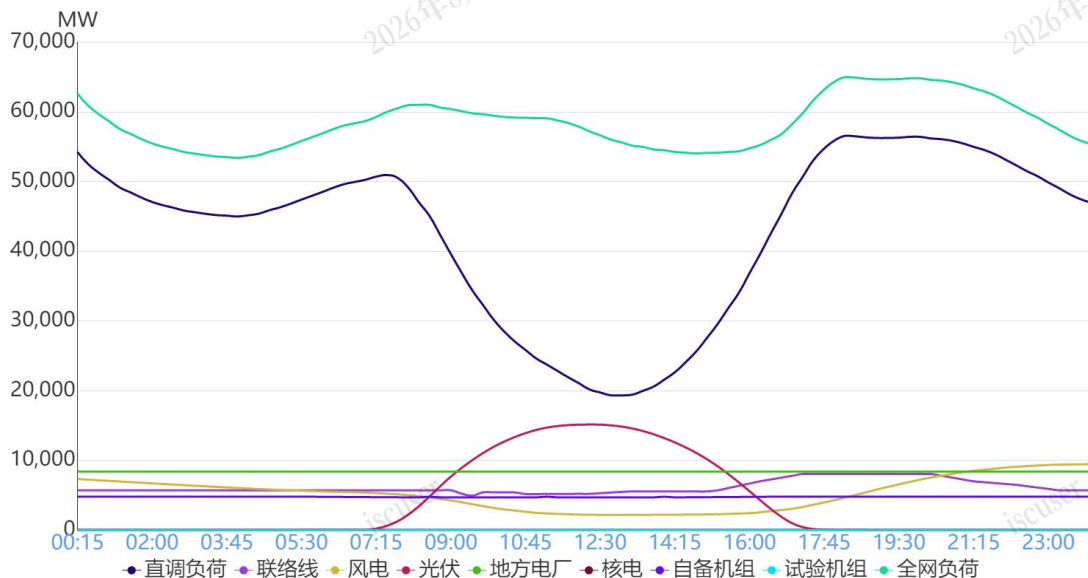
图 1 1月29日负荷及电源出力预测情况
