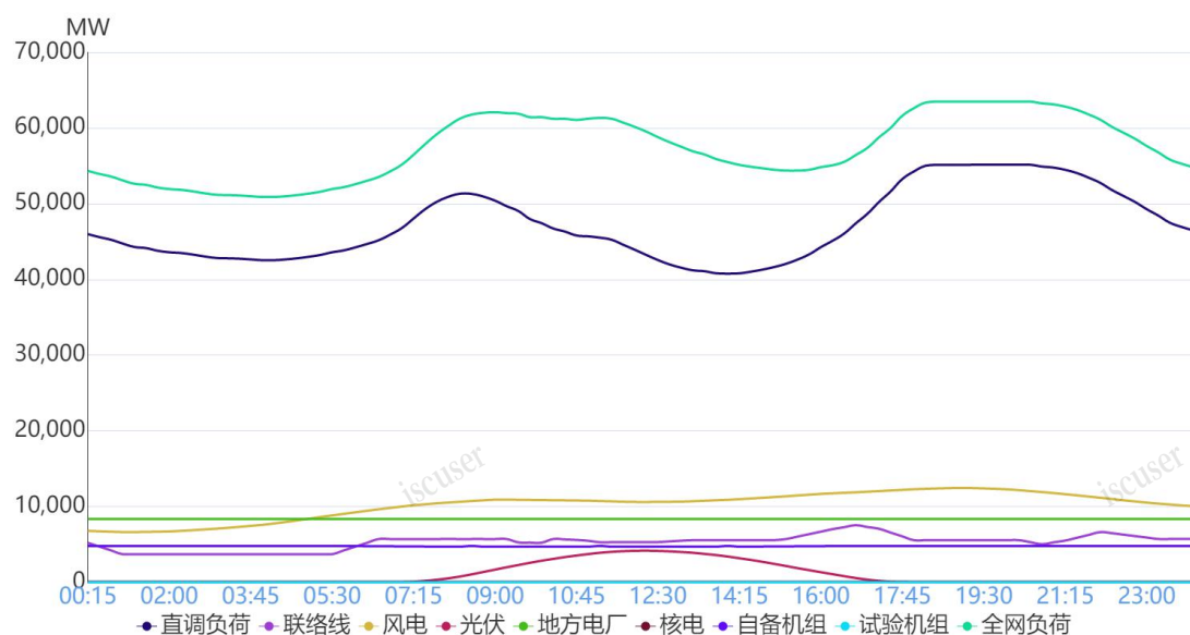
图1 1月31日负荷及电源出力预测情况
