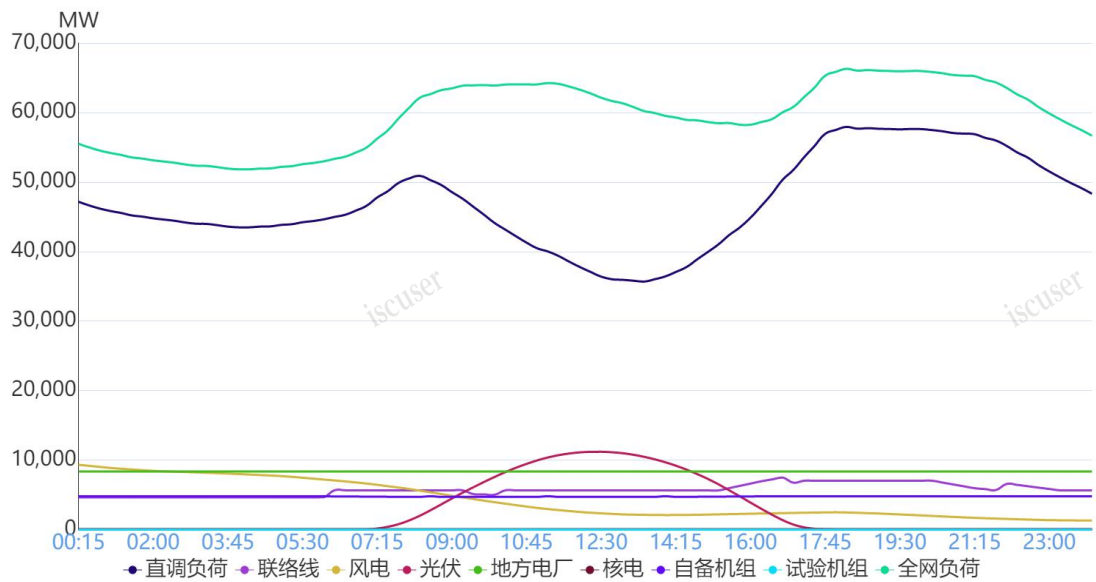
图 1 2 月 1 日负荷及电源出力预测情况
