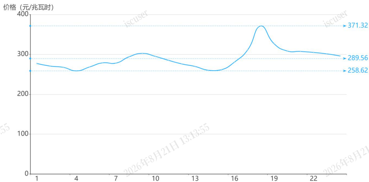
图3 2月1日实时市场用电侧价格
