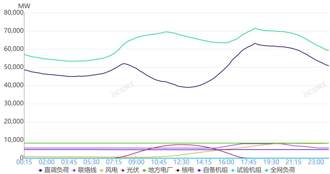
图 1 2 月 2 日负荷及电源出力预测情况
