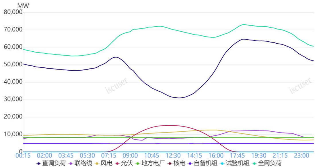
图 1 2 月 3 日负荷及电源出力预测情况
