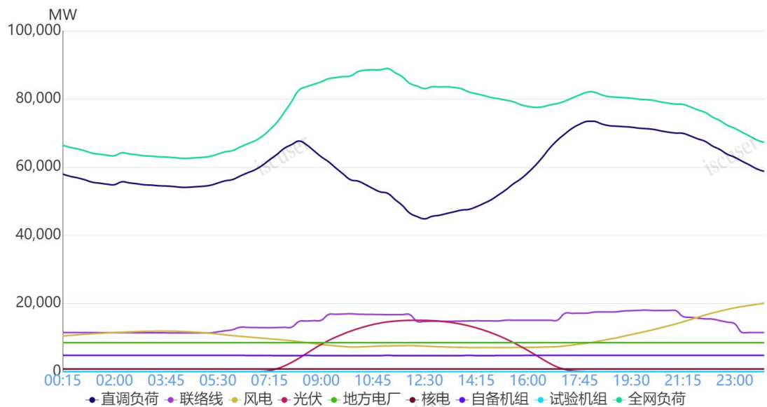
图 1 2 月 6 日负荷及电源出力预测情况
