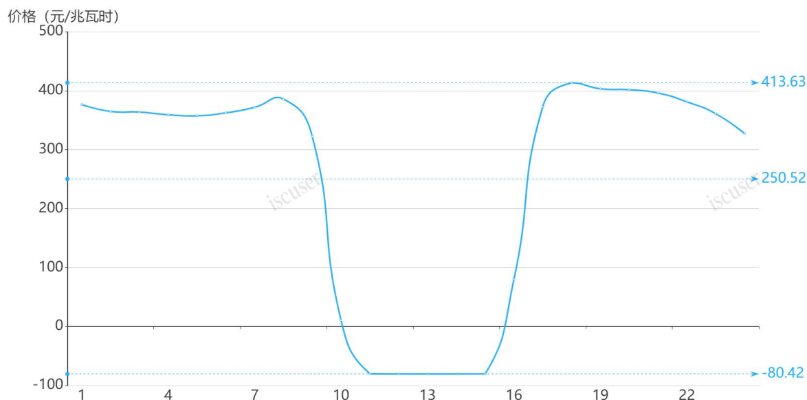
图2 2月9日日前市场用电侧价格
