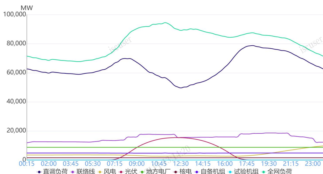
图 1 2月9日负荷及电源出力预测情况
