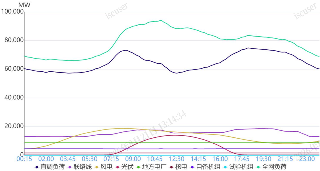
图 1 2月12日负荷及电源出力预测情况
