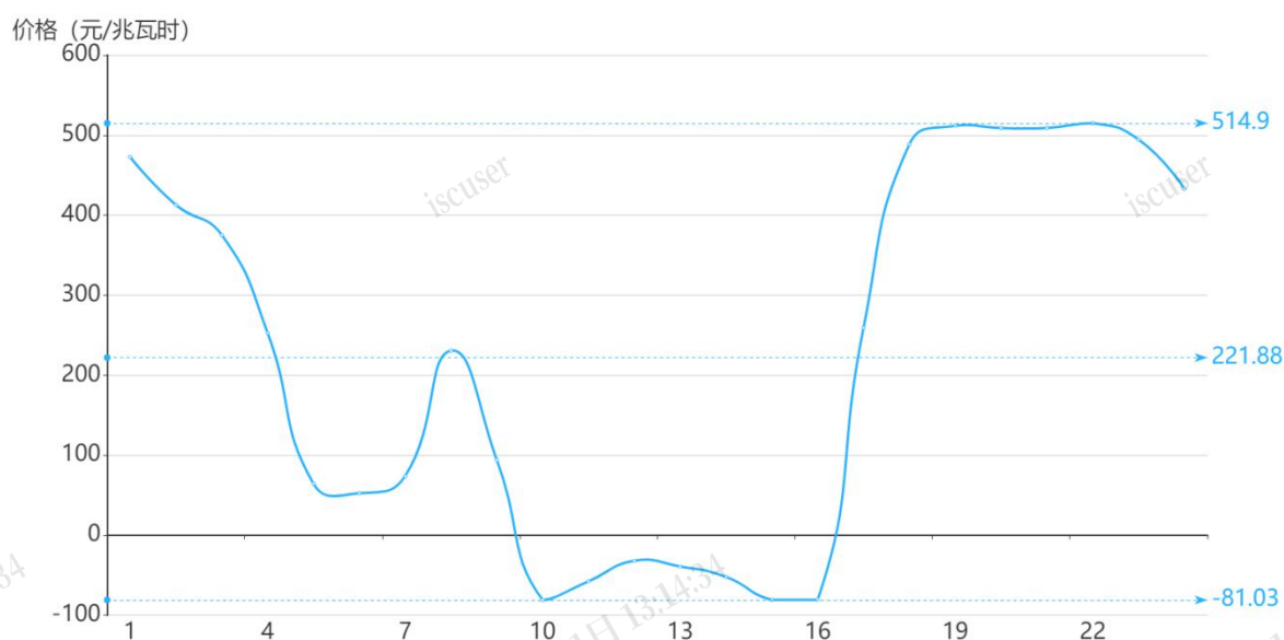
图 2 2 月 12 日日前市场用电侧价格
