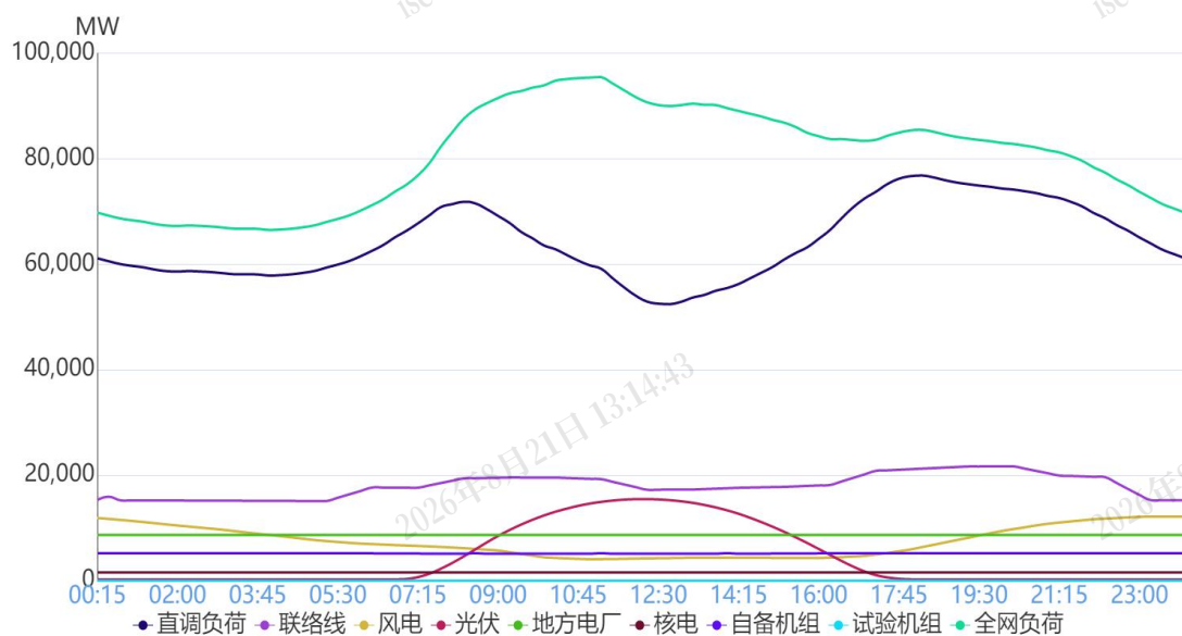
图 1 2月14日负荷及电源出力预测情况
