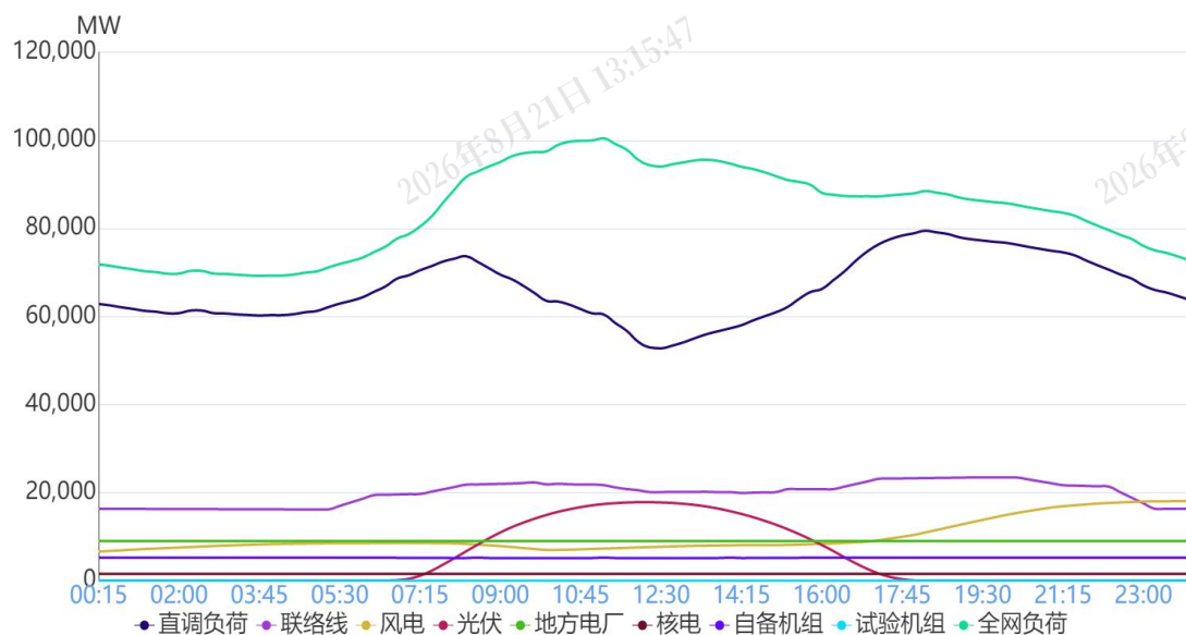
图 1 2月24日负荷及电源出力预测情况
