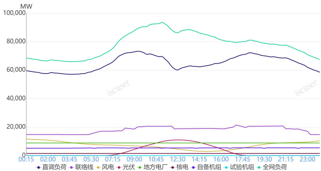
图 1 3 月 1 日负荷及电源出力预测情况
