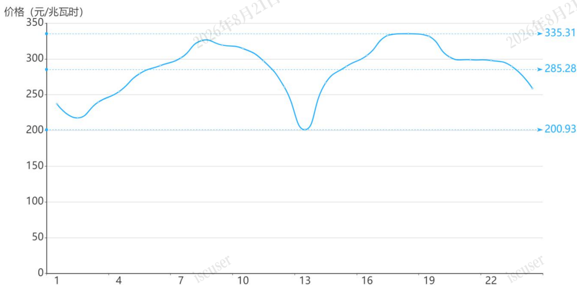
图2 3月1日日前市场用电侧价格
