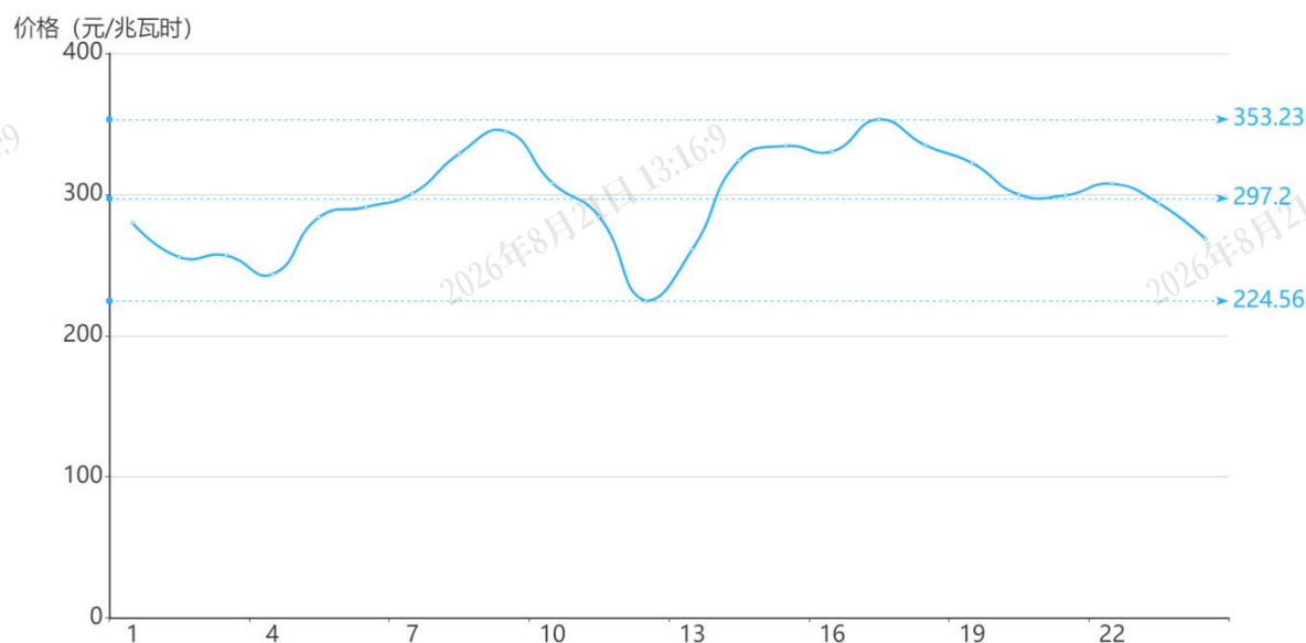
图 3 3 月 1 日实时市场用电侧价格
