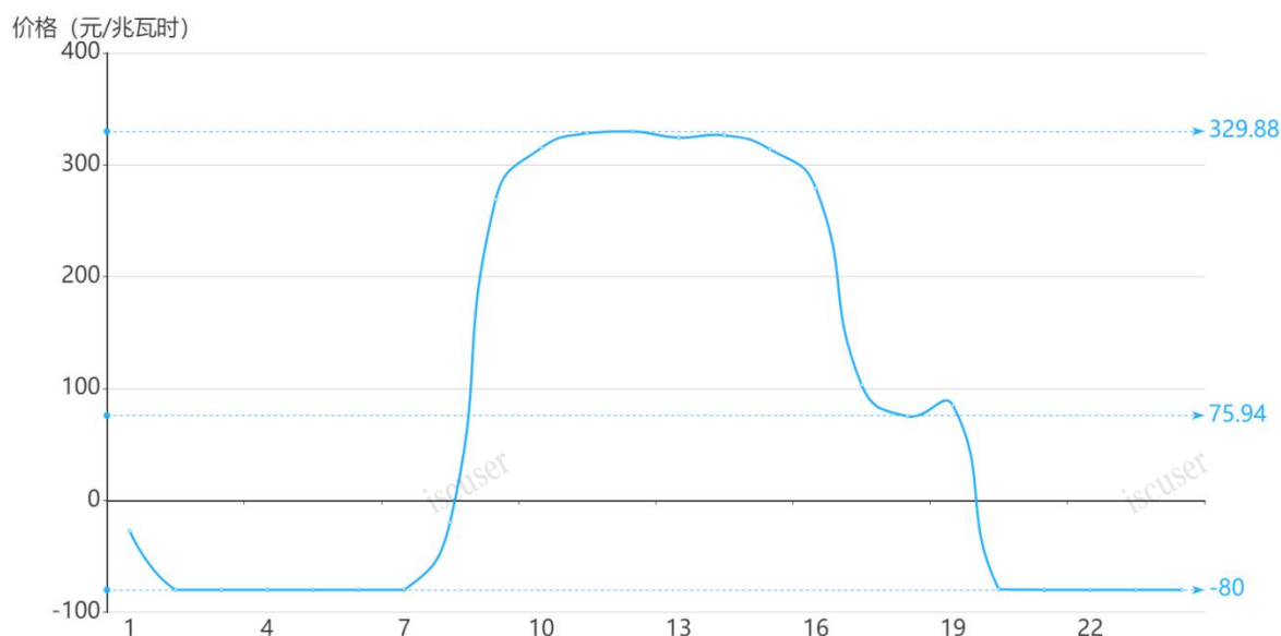
图2 3月2日日前市场用电侧价格
