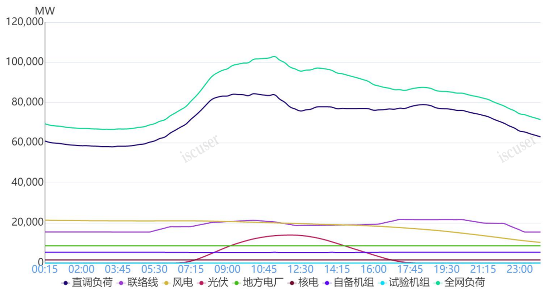
图 1 3 月 3 日负荷及电源出力预测情况
