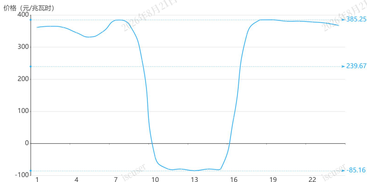
图2 3月6日日前市场用电侧价格
