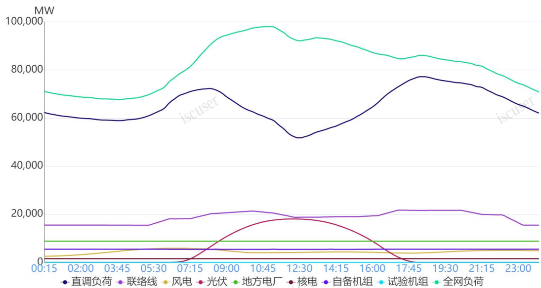
图 1 3 月 6 日负荷及电源出力预测情况
