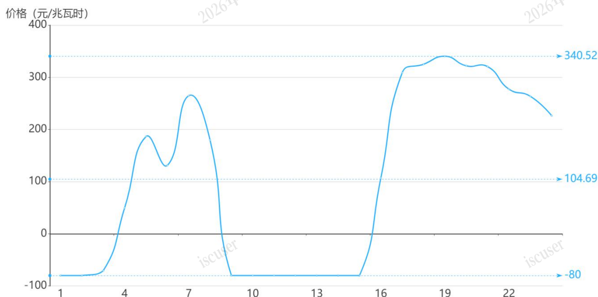
图 3 3 月 10 日实时市场用电侧价格
