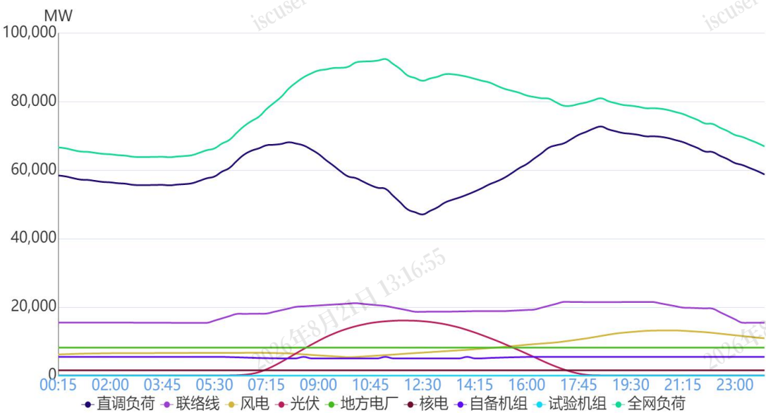
图 1 3月13日负荷及电源出力预测情况
