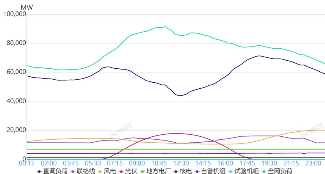
图 1 3月31日负荷及电源出力预测情况
