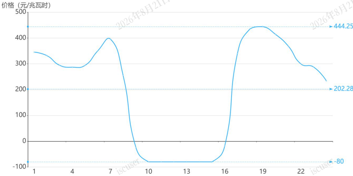
图 2 3 月 31 日日前市场用电侧价格
