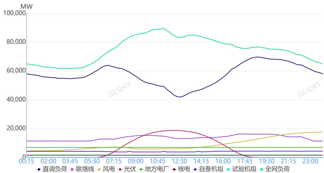
图 1 4 月 3 日负荷及电源出力预测情况
