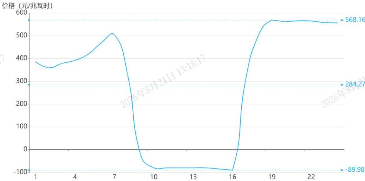
图3 4月2日实时市场用电侧价格
