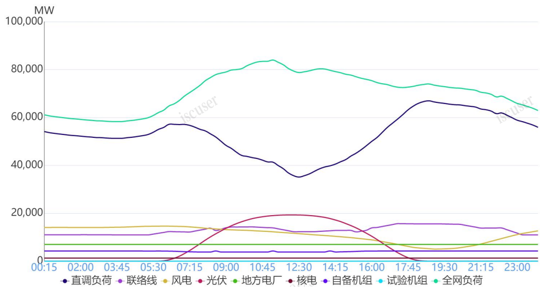
图 1 4 月 5 日负荷及电源出力预测情况
