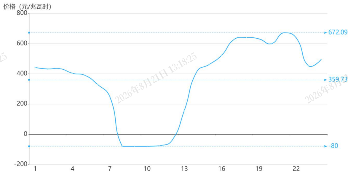
图3 4月4日实时市场用电侧价格
