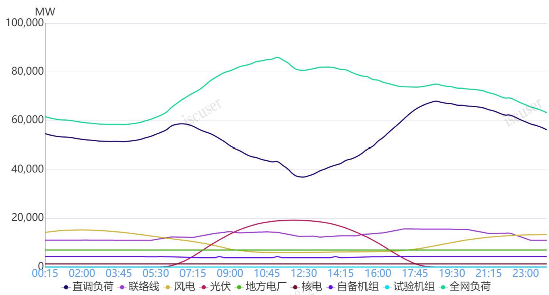
图 1 4 月 6 日负荷及电源出力预测情况
