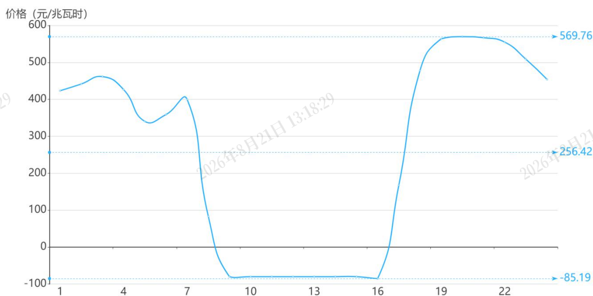
图 3 4月5日实时市场用电侧价格
