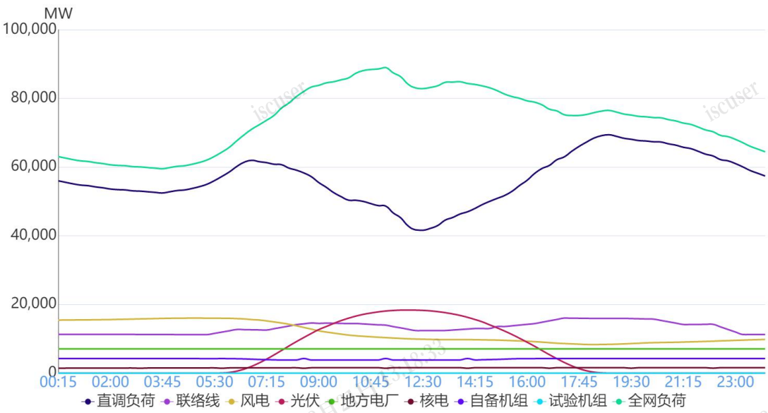
图 1 4月7日负荷及电源出力预测情况
