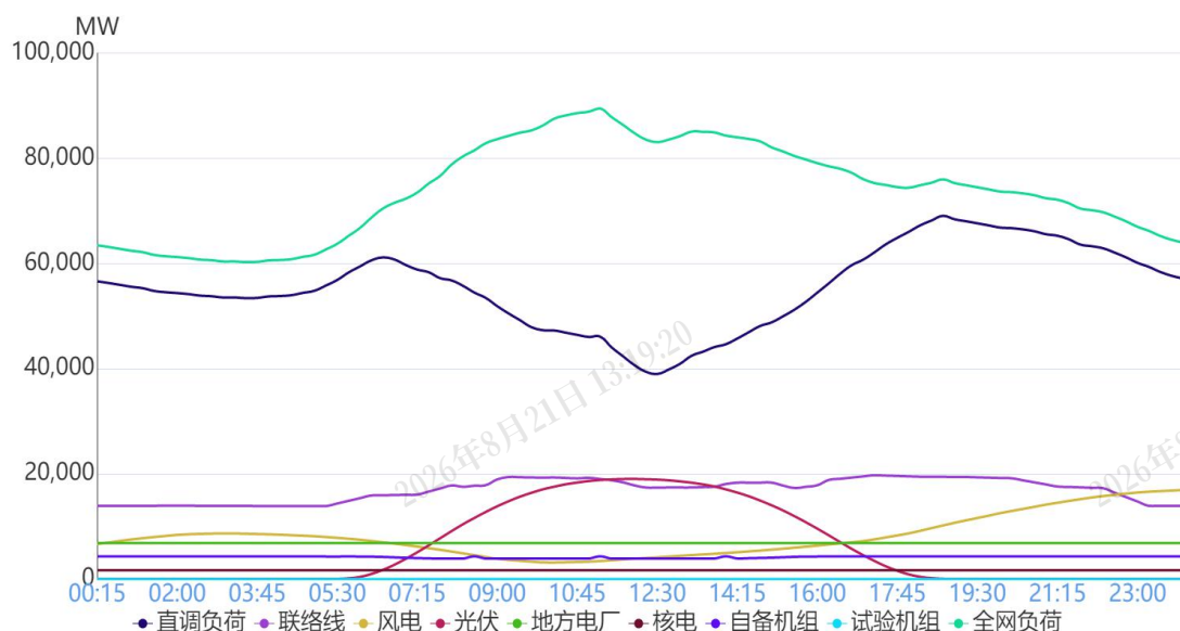
图1 4月15日负荷及电源出力预测情况
