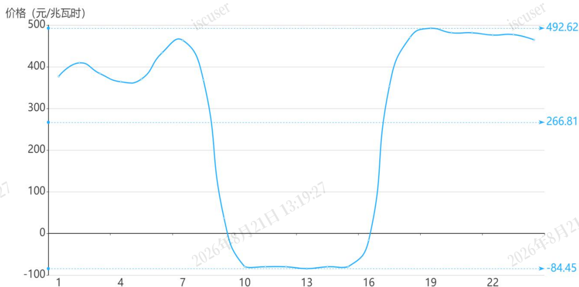
图2 4月17日日前市场用电侧价格
