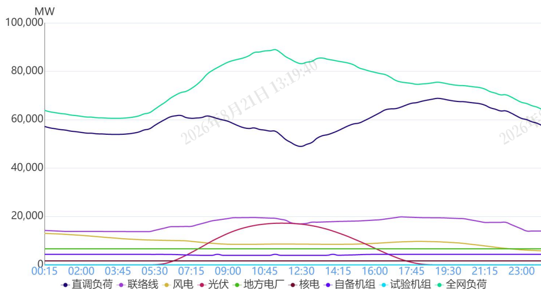
图 1 4月21日负荷及电源出力预测情况
