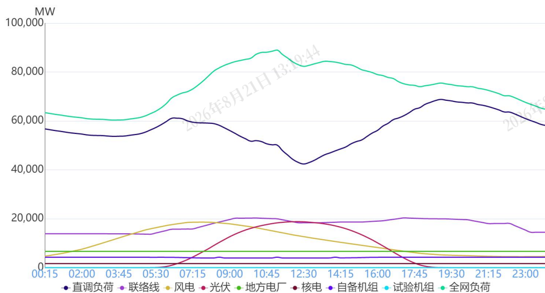
图 1 4月22日负荷及电源出力预测情况
